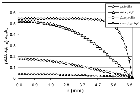
شکل ۷- تغییرات رطوبت از مرکز به سطح دانه با رطوبت اولیه 0.54/62\% ، کل 70^{\circ}\text{C} و ضریب پخش رطوبت (7/5 \times 10^{-11} \text{ m}^2/\text{s})
