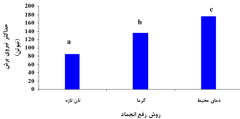
نمودار 4 رابطه روش رفع انجماد نان های لواش و حداکثر نیروی برش میانیگین هایی که با حروف مختلف نشان داده شده اند، با آزمون توکی در سطح \alpha=0/05 با یکدیگر اختلاف معنی دار دارند.
