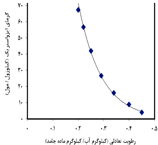
شکل ۵ تغییرات انرژی پیوندی در مقابل افزایش میزان رطوبت
