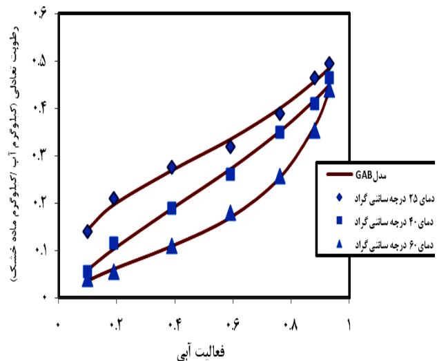
شکل ۳ برازش داده های تجربی با مدل گب در دماهای مختلف
