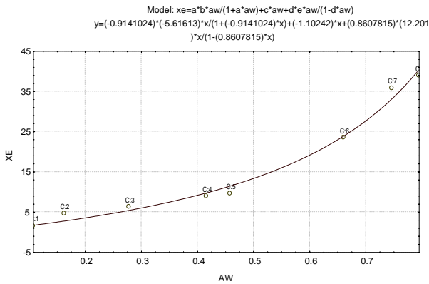
شکل ۷ برازش مدل آرسی وات با داده های آزمایش در دمای ۷۰ درجه سانتی گراد
