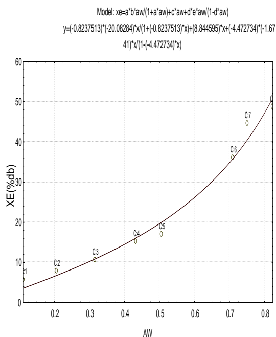
شکل ۴ برآزش مدل آرسی وات با داده‌های آزمایش در در دمای ۴۰ درجه سانتی‌گراد
