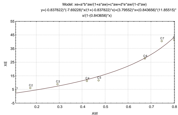
شکل ۶ برازش مدل آرسی وات با داده های آزمایش در دمای ۶۰ درجه سانتی گراد
