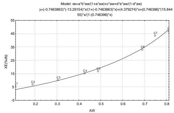
شکل ۵ برازش مدل آرسی وات با داده های آزمایش در دمای ۵۰ درجه سانتی گراد
