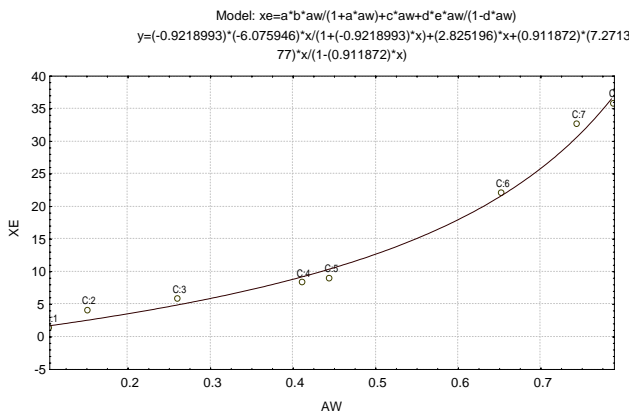
شکل ۸ برازش مدل آرسی وات با داده های آزمایش در دمای ۸۰ درجه سانتی گراد
