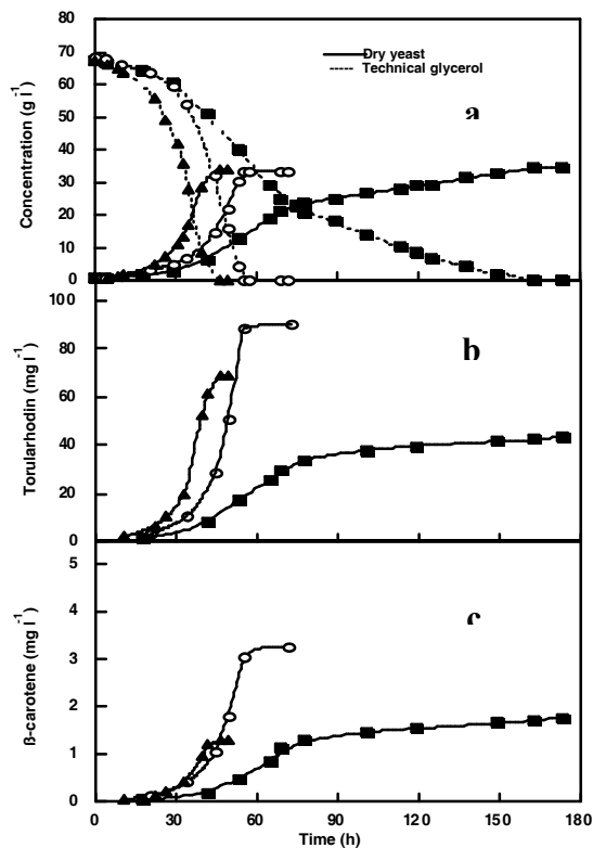
شکل ۱- کیتیک رشد مخمر (a) و تولید تورولا رودین (b) و بتا کاروتن (c) ( میلی گرم در لیتر) توسط اسپوروبولومیسز رو بریموس بر روی غلظتهای مختلف سولفات آمونیوم. pH و درجه حرارت بترتیب در ۶ و ۲۳ °C ثابت نگهداری شد. ■ ۳ گرم در لیتر، ○ ۲۰ گرم در لیتر و ▲ ۳۰ گرم در لیتر.
