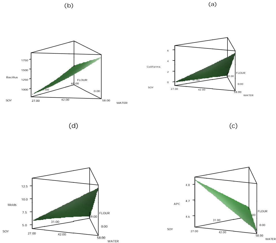
شکل ۲ نمودارهای سطح مخلوط مربوط به شمارش کلی فرم (a)، باسیلوس (b)، شمارش کلی (c)، کپک و مخمر (d)، در نقطه بهینه فرایند (سرعت چرخش ماریپیج ۱۰ دور بر دقیقه و دمای آب سیرکولاسیون ۳۵ درجه سانتی گراد).
